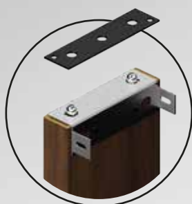
inserti esterni già montati
